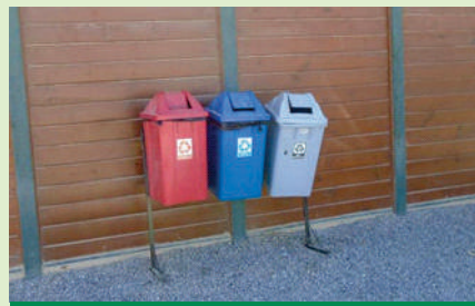
Exemplo de medida do Plano Ambiental da Construção (PAC): gestão de resíduos sólidos – coletores seletivos espalhados no canteiro de obras, contendo placas de identificação por tipo de resíduo e padrões de cores
